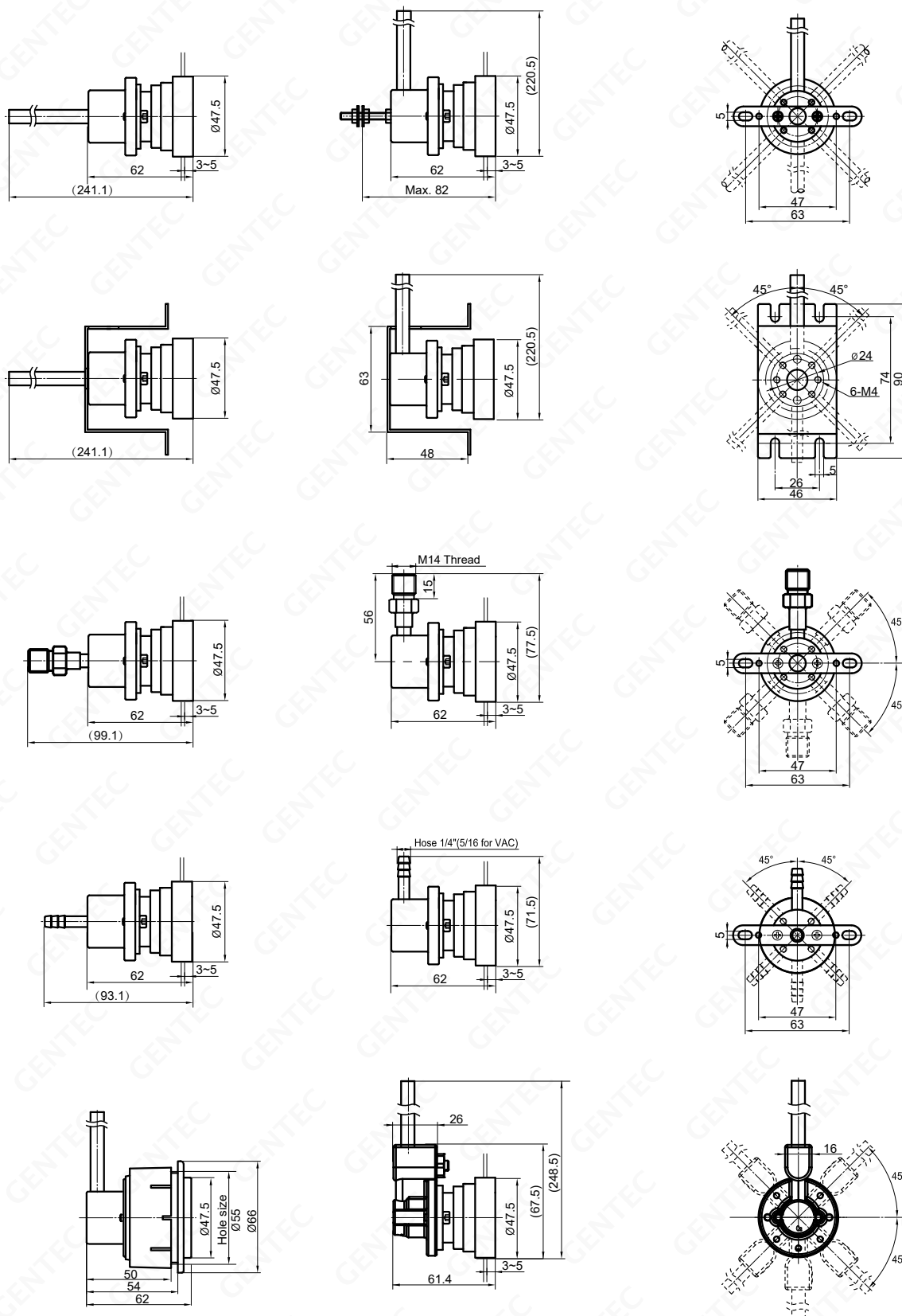
平面压盖式尺寸图 Dimensions (mm)
