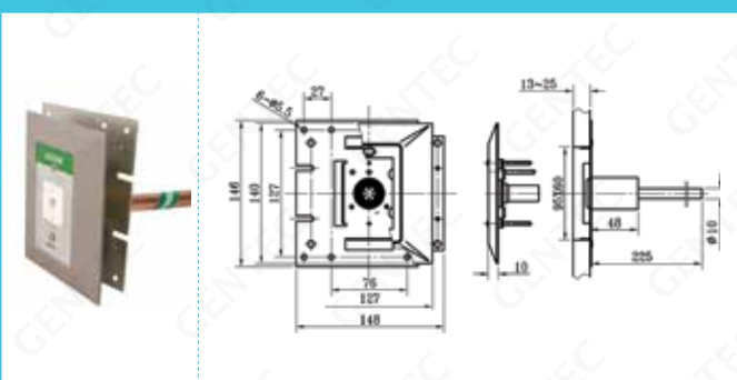
覆壁式 180° 焊接铜管进气
