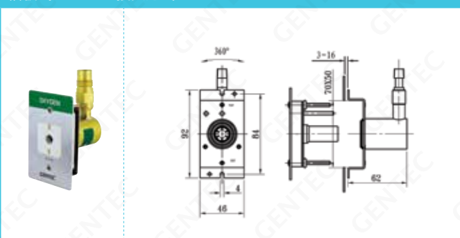
覆壁式 90° 焊接铜管进气
